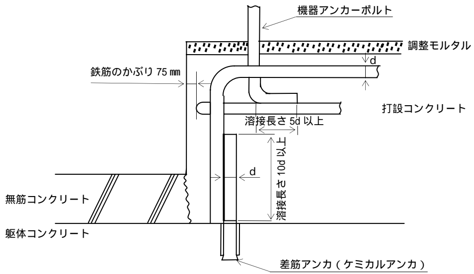
図2 静荷重形基礎要領図
