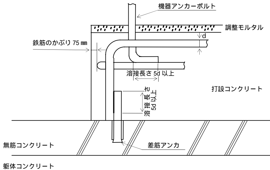
図3 軽荷重形基礎要領図
