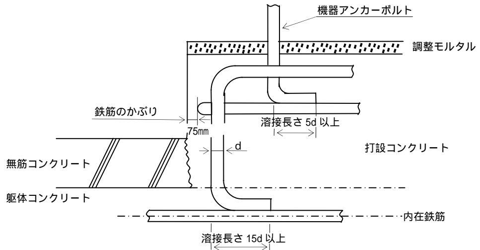
図 1 重荷重形基礎要領図
